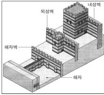
▲ 성벽 구조도
