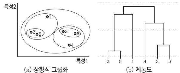
&lt;그림 2&gt; 계층법의 예
