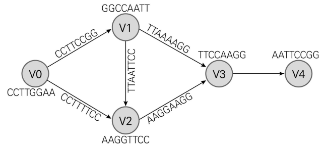
&lt;그림 2&gt; 정점 5개로 구성된 그래프
