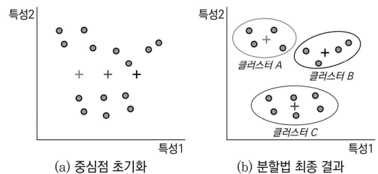
<그림 1> 분할법의 예
