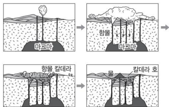
함몰 칼데라의 형성 과정
